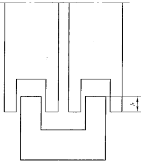
图 2 左右推拉窗
